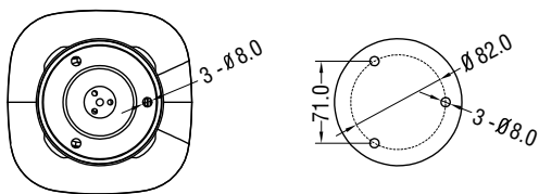
Vista Inferior (base)
