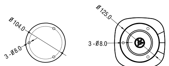
Vista Inferior (base)
